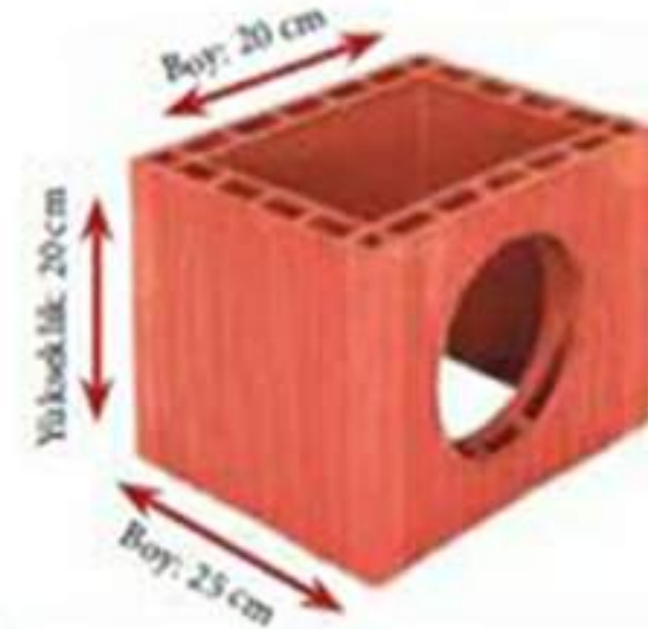
Kare Delikli Baca Tuğla
