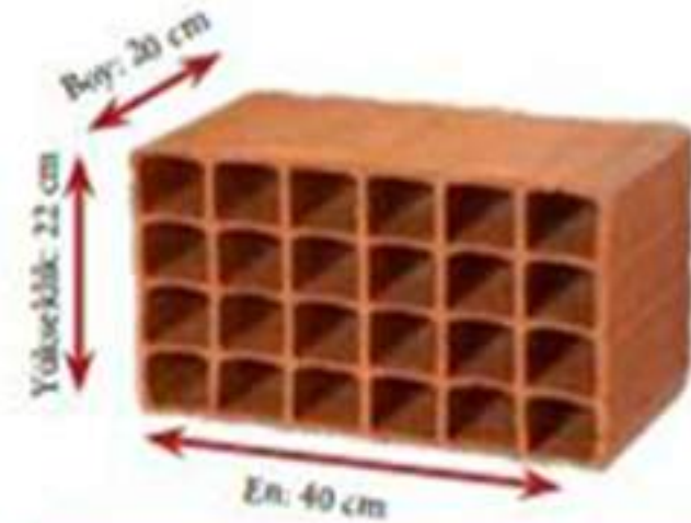
22,5'lik Asmolen Tuğla
