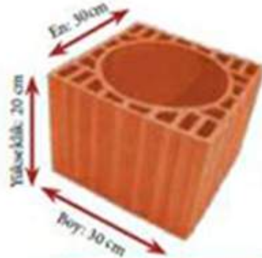
Kalorifer Bacası
