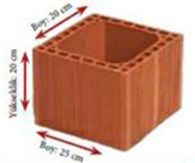
Kare Baca
