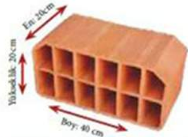
20'lik Asmolen Tuğla
