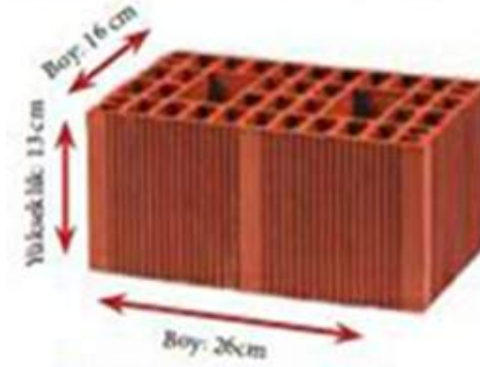
Yığma Tuğla
