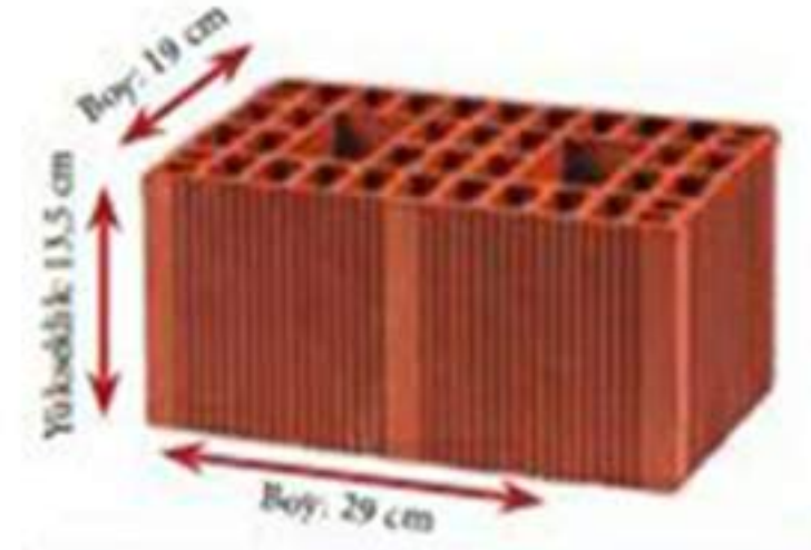
Büyük Yığma Tuğla
