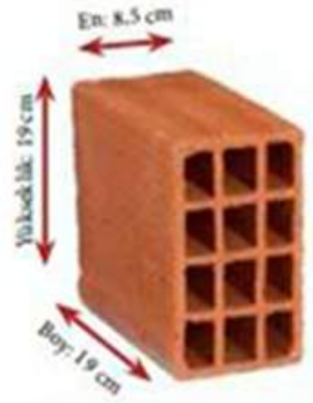
8,5'lik Tuğla
