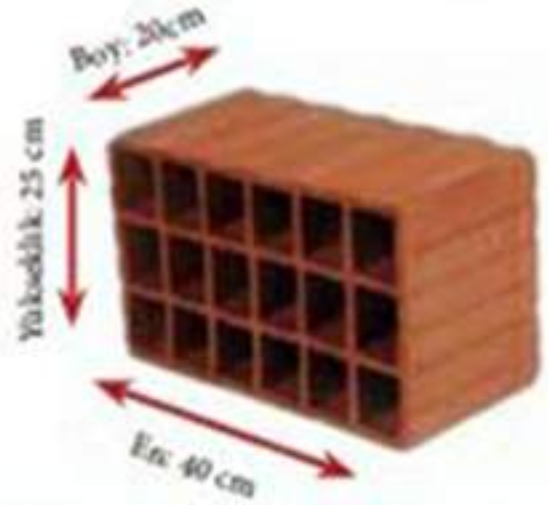
25'lik Asmolen Tuğla
