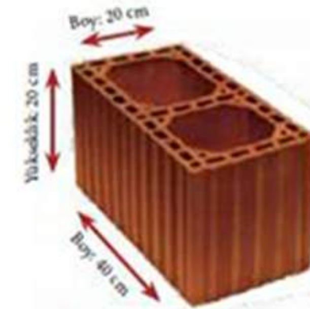
Çift Şön Tuğla
